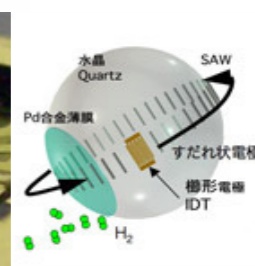
ボール SAW 水素ガスセンサの構造と原理
